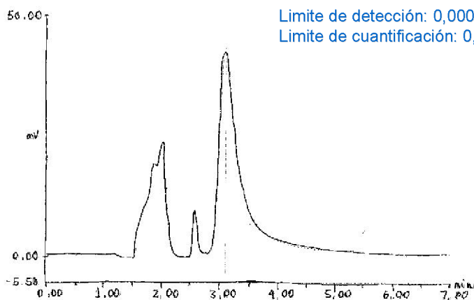
Cromatograma HPLC, de Clenbuterol en hígado de cerdo
